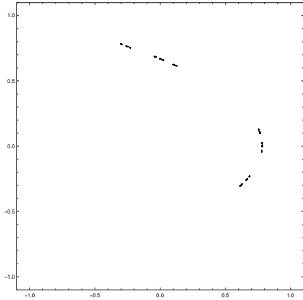
(a) A six times period-doubling renormalizable Hénon map.
